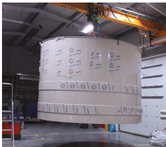
Kruhová nádrž PP (objem 45m 3 )
